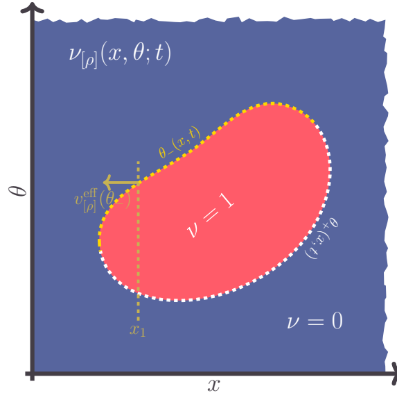
FIGURE III .2 – Schéma de l'évolution du facteur d'occupation \nu(x, \theta, t) dans la limite \gamma \rightarrow 0 . Initialement rectangulaire et homogène, la distribution forme une mer de Fermi délimitée par \theta_{\pm}(x, t) : rouge \nu = 1 , blue \nu = 0 .
