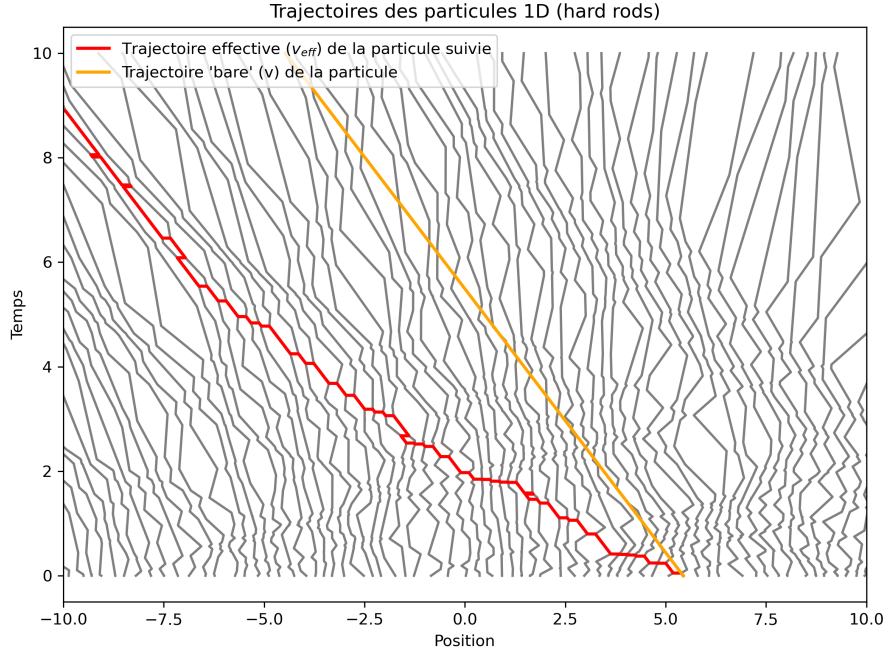
FIGURE III .1 – Trajectoires des particules d'un gaz de barres dures en 1D. Les lignes noires représentent les particules individuelles, la ligne rouge la trajectoire effective (vitesse GHD ) de la particule suivie, et la ligne orange la trajectoire si la particule conservait sa vitesse initiale (bare velocity). Le graphique a été généré en Python.
